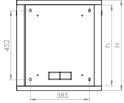
Arka Görünüş
