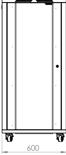
Ön Görünüş
