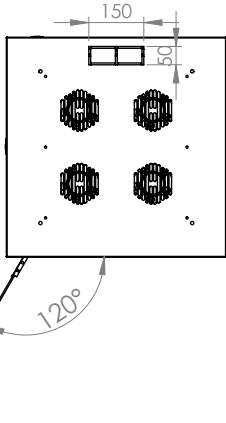
Üst Görünüş
