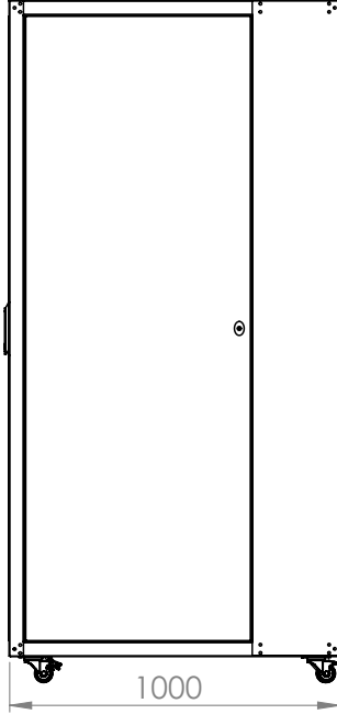
Yan Görünüş
