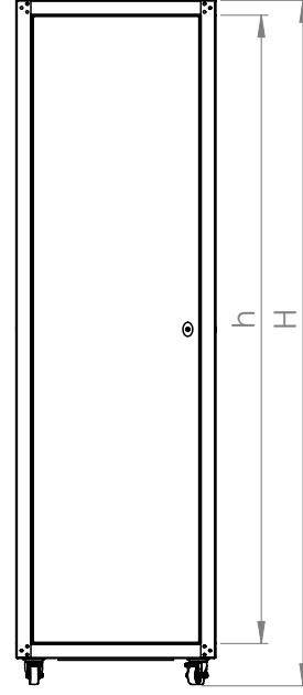
Arka Görünüş
