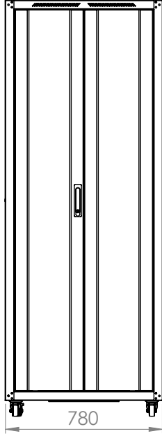
Ön Görünüş
