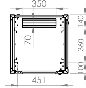
Detay Görünüş
