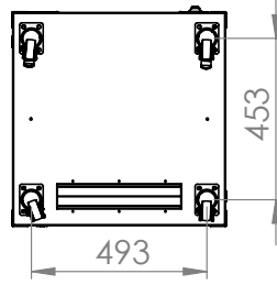
Alt Görünüş
