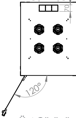
Üst Görünüş
