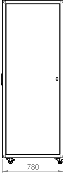
Yan Görünüş
