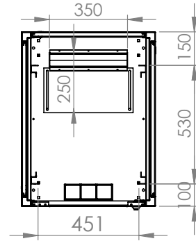
Detay Görünüş
