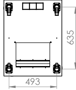
Alt Görünüş
