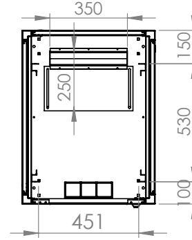
Detay Görünüş
