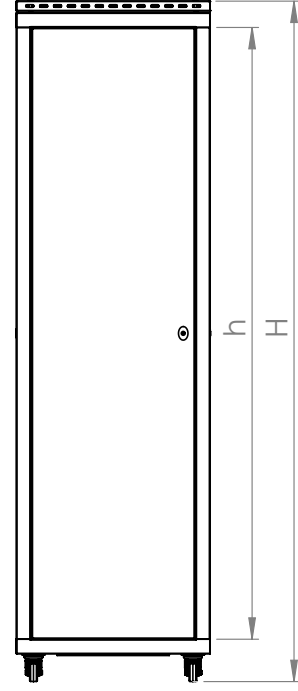
Arka Görünüş
