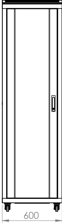
Ön Görünüş
